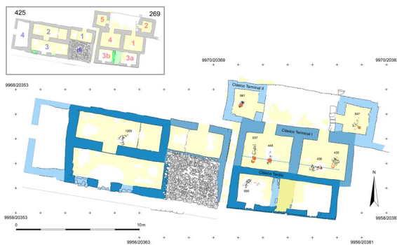
Figura 4: Los edificios 269 (derecha) y 425 (izquierda), con los últimos pisos dentro de los cuartos y los entierros del Clásico Terminal (dibujo: Proyecto Arqueológico Dzehkabtún).
